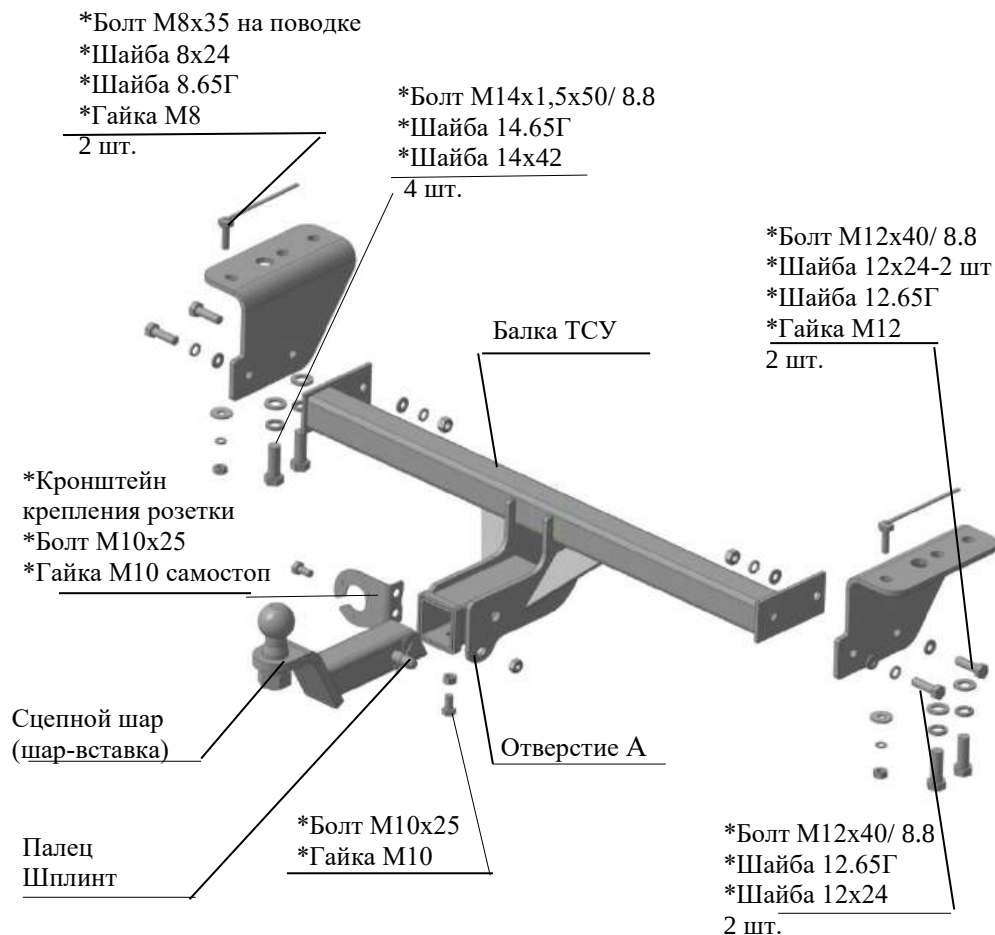
Рис.1 Тягово-сцепное устройство ТСУ 8161.
